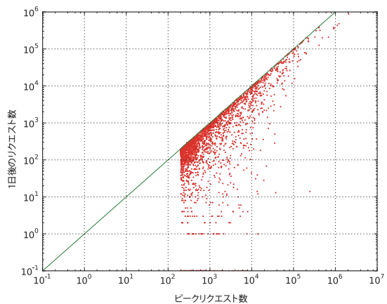
図-5 コンテンツごとのリクエスト数の変化(1日後)
